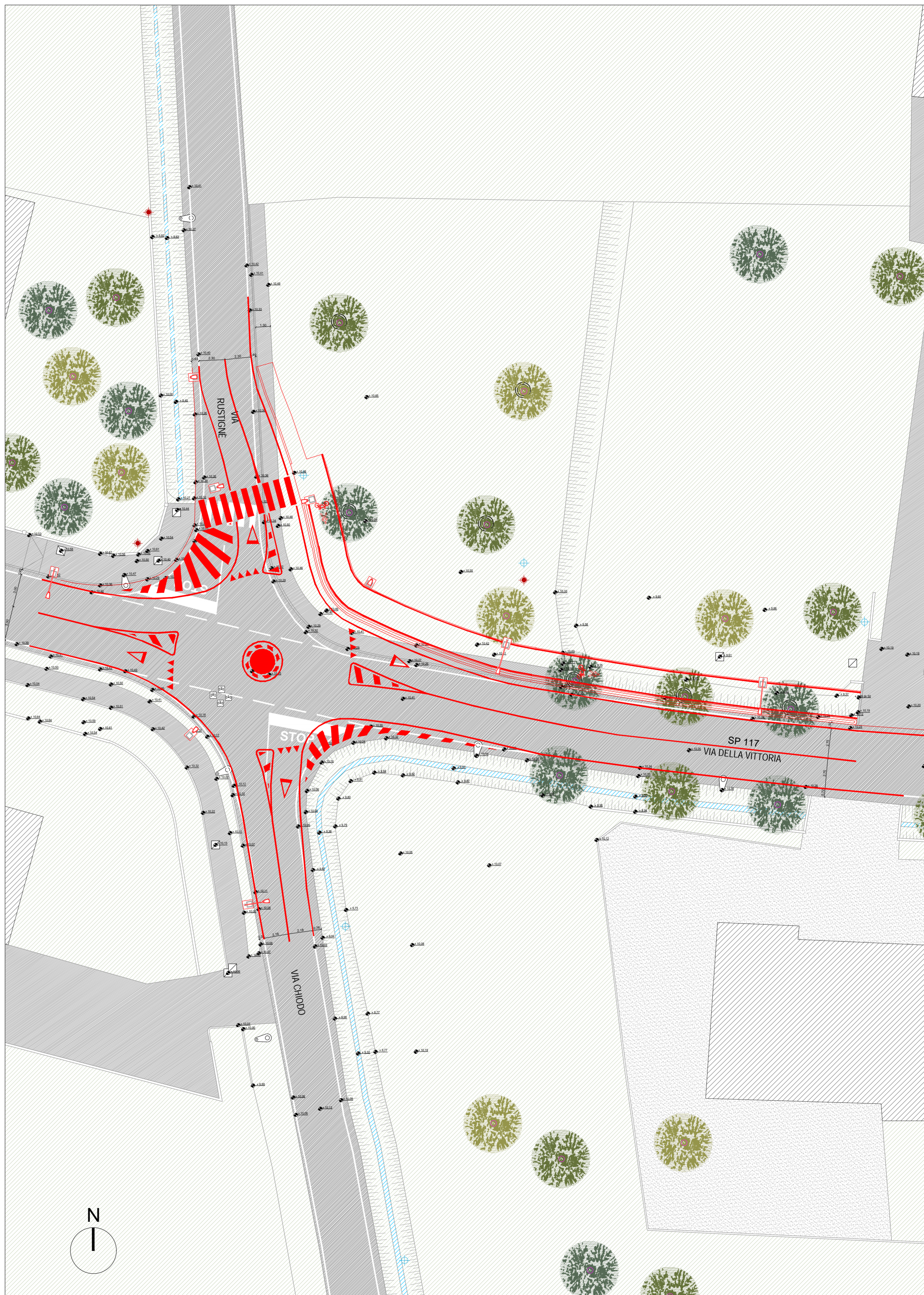
Planimetria stato di comparativo - scala: 1:200
